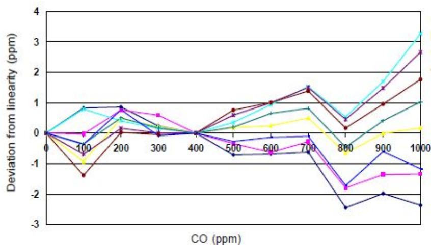
图4 1000ppm线性度
